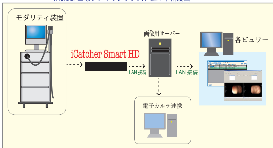
iHolder 画像ファイリングシステム基本構成図
